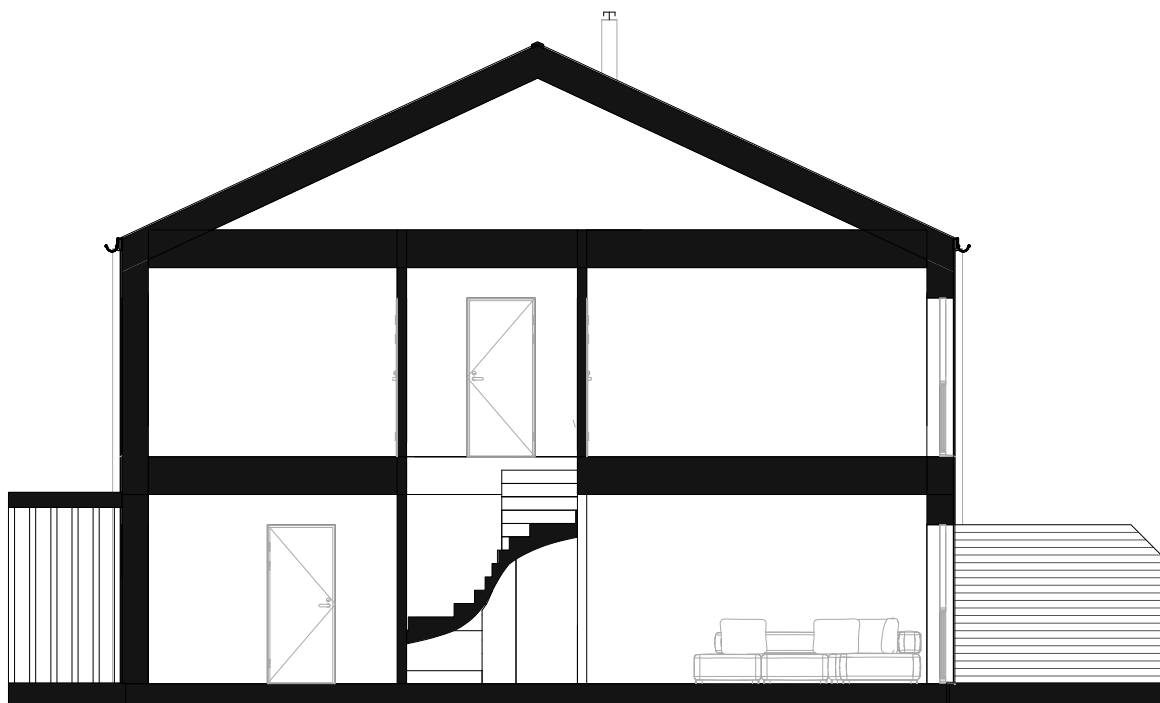
S2 M 1 : 100
