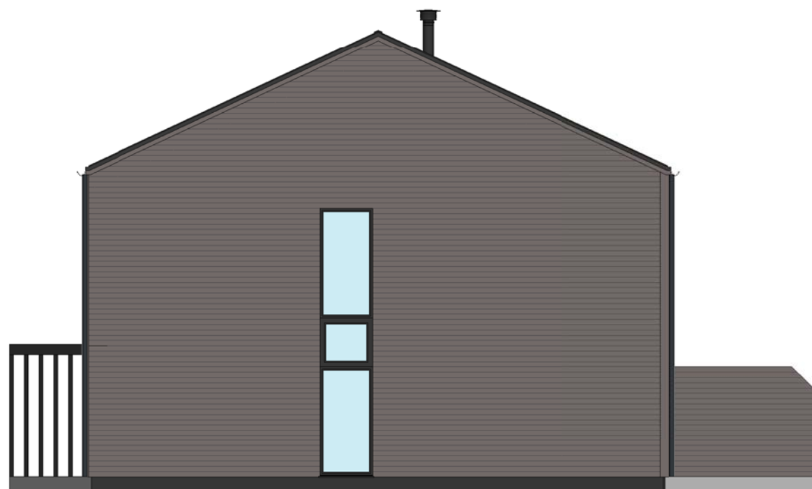
SØR M 1 : 100
